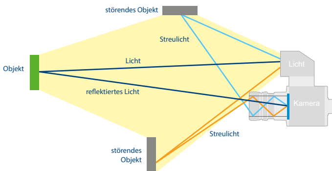
Abbildung 5 - Streulicht
