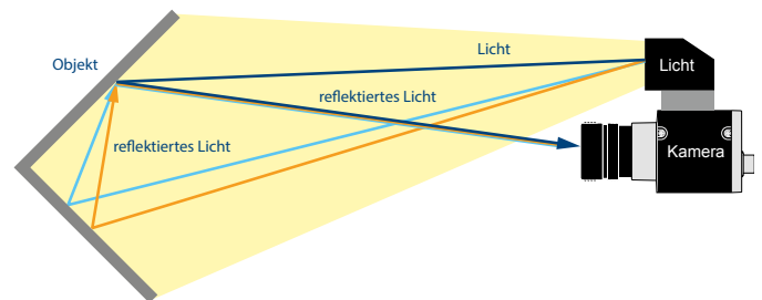
Abbildung 4 - Mehrfach-Reflexion
